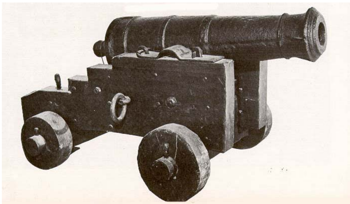
1.47. Brodski top sa lafetom iz XVIII i XIX vijeka.
