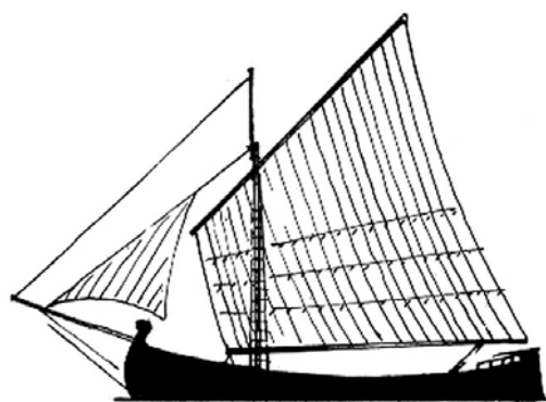
Bracera — slična je gajeti, ali većih dimenzija. Osobito se ističe većom širinom trupa u odnosu prema dužini, tj. nije tako vitka kao gajeta. Obično vodi sa sobom manji čamac. Nosivost 10—40 tona. Bracera je na našoj obali vrlo rasprostranjen tip broda
