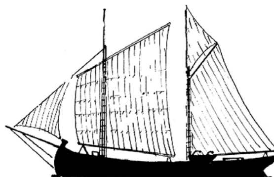
Trabakul — veći obalni jedrenjak, koji katkada prelazi i na drugu obalu Jadrana. Sličan je braceri, ali je većih dimenzija. Obično vuče sa sobom čamac. Posada mu se sastoji od 4—5 osoba, a nosivost mu je 40—140 tona
